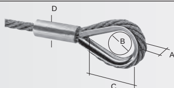
Capocorda con redancia e boccia a pressione Loop with thimble and press sleeve
