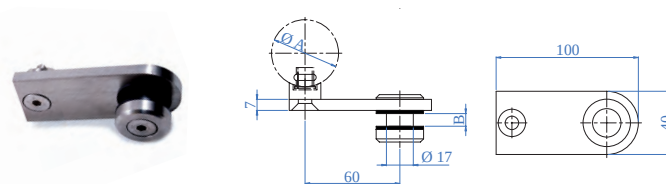
3 pezzi : un braccio, 1 supporto circolare per vetro e un adattatore per tubo 3 pieces: one arm, 1 round clamp for glass, and one tube adapter
