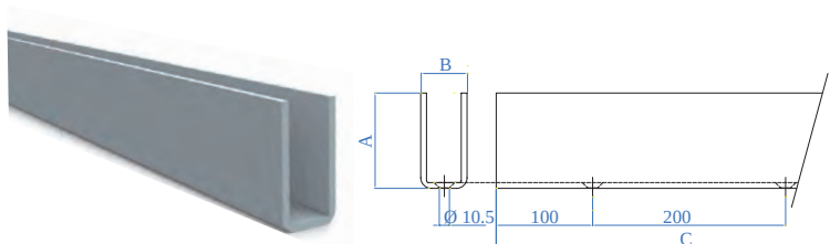
Pre-forato e galvanizzato - Pre-drilled and galvanized
