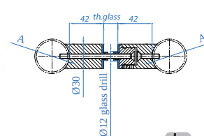
Supporto vetro doppio Double glass support
