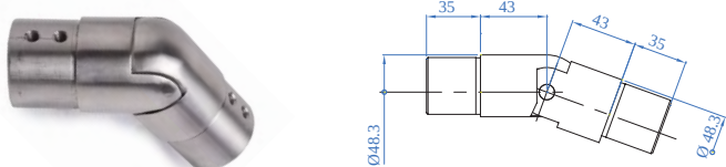
Raccordo snodato 25-55° verso il basso Downward pivotable connector, 25-55°
