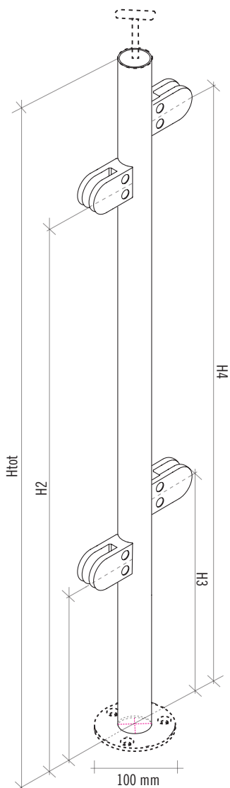
Fisso - Fixed
