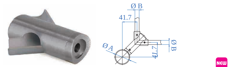
SUPPORTI TONDINO AD ANGOLO ANGLE ROUND BAR HOLDERS
