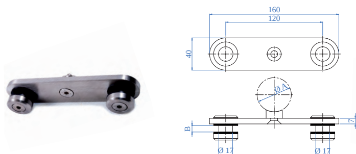
4 pezzi : un braccio, 2 morsetti circolari per vetro e un adattatore per tubo 4 pieces: one arm, 2 round clamps for glass, and one tube adapter
