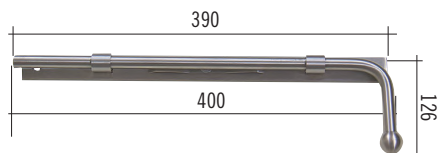
Chiavistello autobloccante, VA-gate latch self-locking, Ø 14 x 450 mm Ø 14 x 450 mm
